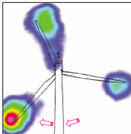
Bild 18: violett rot, Ort der stärksten Schallemission, nach van den Berg [9]
